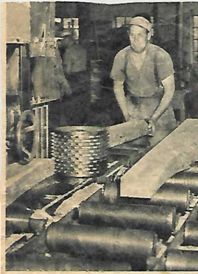
GUSTAV SKOOG delar upp virket i stavämnen.
